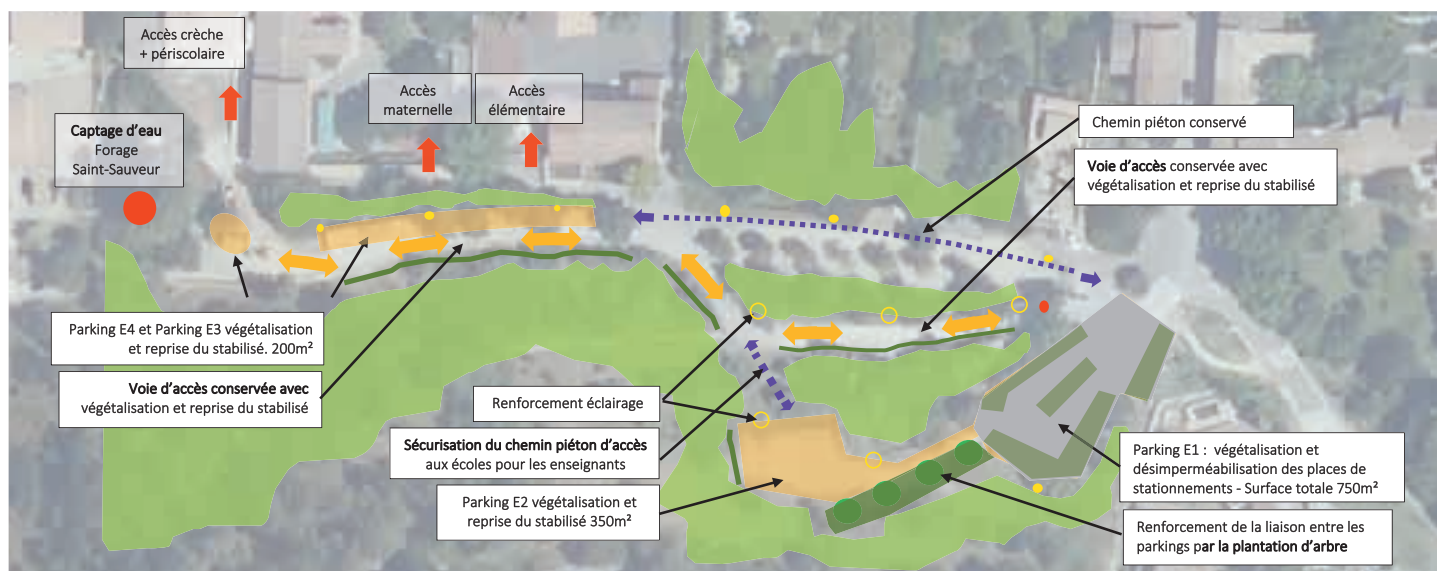
Exemple de parking végétalisé
